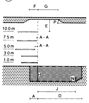
8 Longitudinal section
